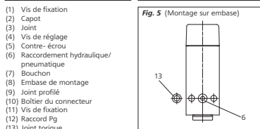
(1) Vis de fixation (2) Capot (3) Joint (4) Vis de réglage (5) Contre-écrou (6) Raccordement hydraulique/pneumatique (7) Bouchon (8) Embase de montage (9) Joint profilé (10) Boîtier du connecteur (11) Vis de fixation (12) Raccord Pg (13) Joint torique
