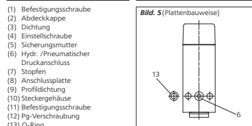
(1) Befestigungsschraube (2) Abdeckkappe (3) Dichtung (4) Einstellschraube (5) Sicherungsmutter (6) Hydr./Pneumatischer Druckschluss (7) Stopfen (8) Anschlussplatte (9) Profildichtung (10) Steckergehäuse (11) Befestigungsschraube (12) Pg-Verschraubung (13) O-Ring
